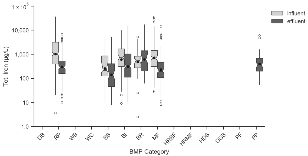
Figure 5-9. Box Plots of Influent/Effluent Total Iron (µg/L).
