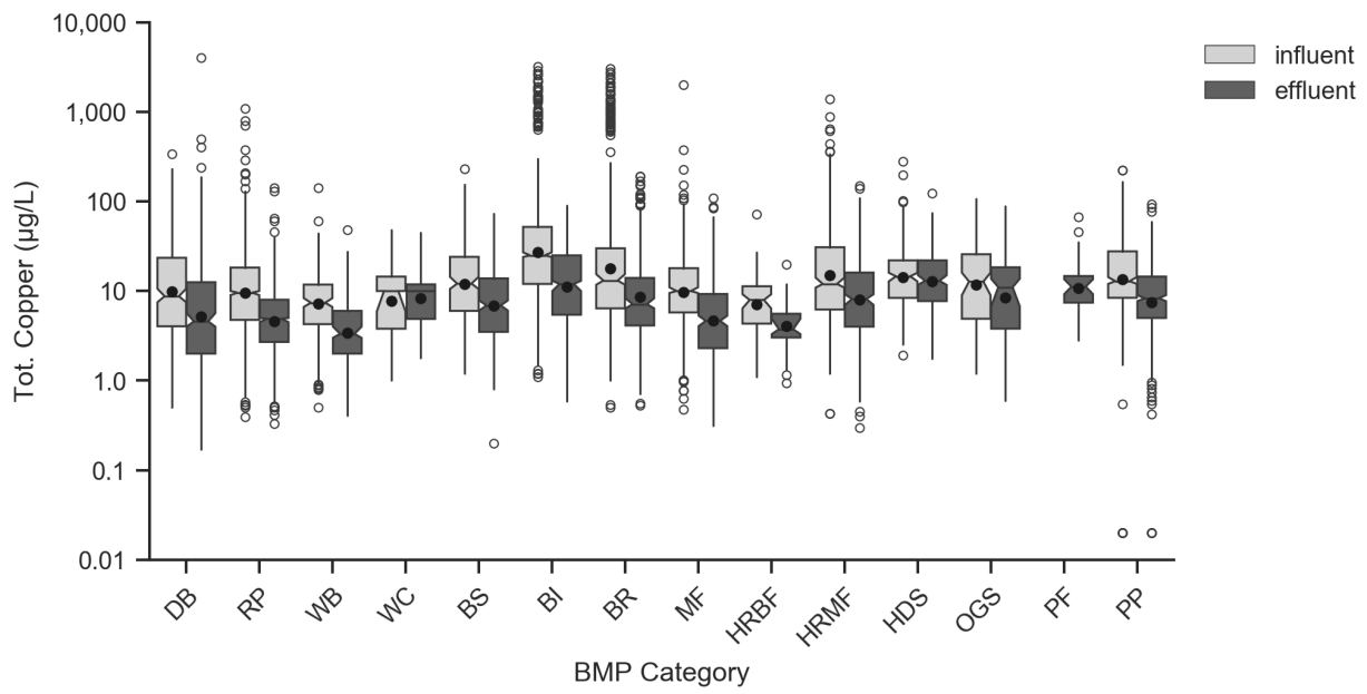
Figure 5-7. Box Plots of Influent/Effluent Total Copper (µg/L).
